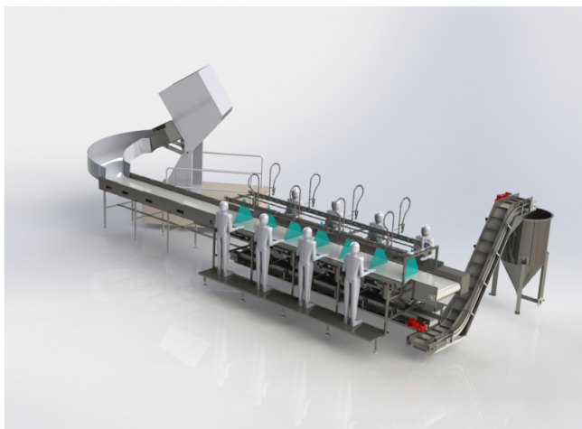
Renderizado de Línea de producción de Gaitech diseñada con SOLIDWORKS PhotoView360
