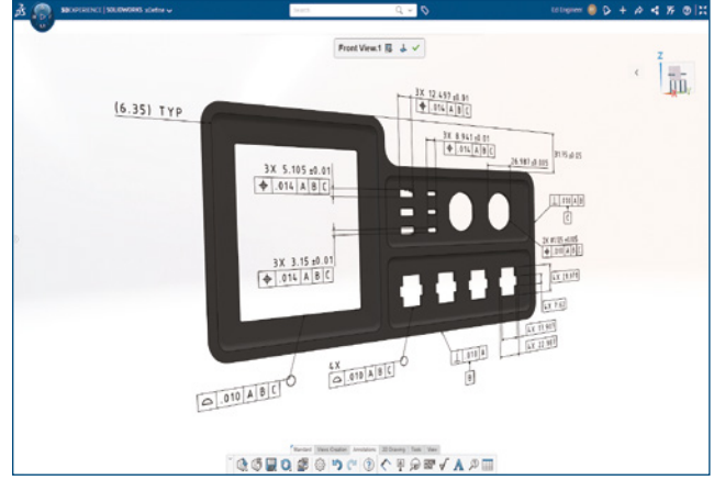
Tasarım gereksinimlerini 3D olarak hızlı ve sezgisel bir şekilde tanımlama.
