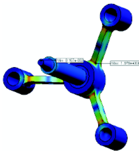
응력 해석
