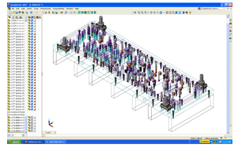
Wireframe lower die set
