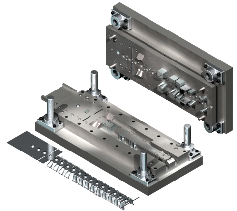
Bermo Inc. die design
